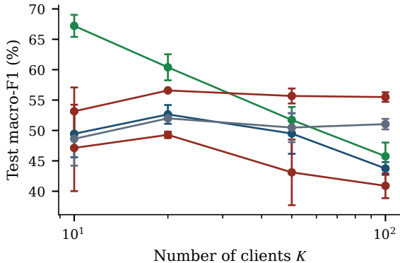
CICIoT2023
