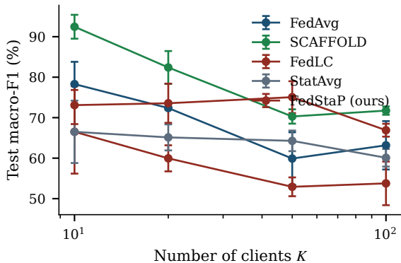
Edge-IIoTset
