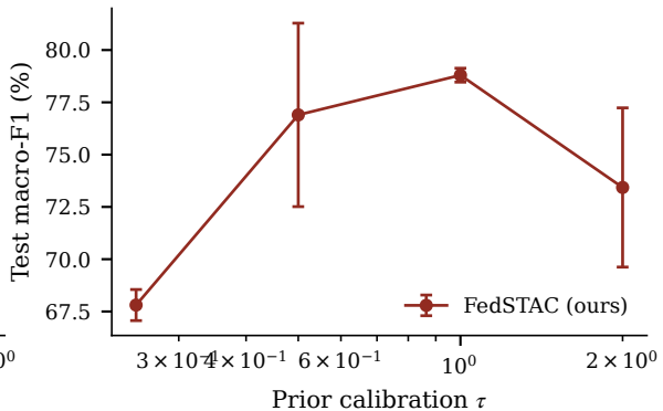
Edge-IIoTset
