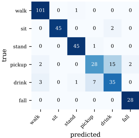
CNN, validation participants
