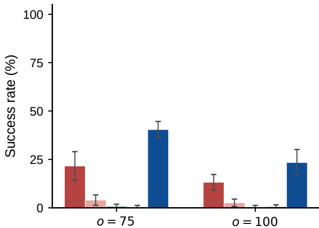
PushT
