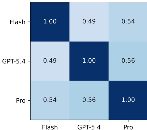
ALFWORLD - No-Skill
