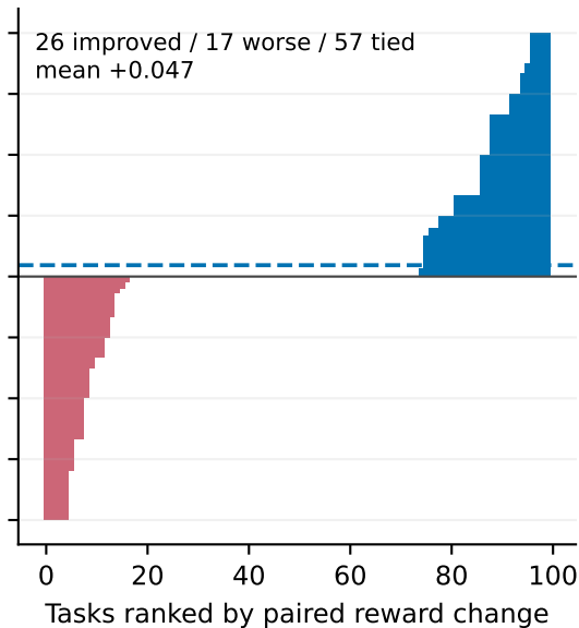
GPT-5.4
