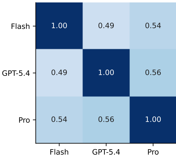
ALFWORLD - No-Skill
