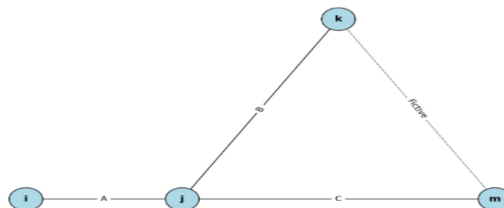
Exemple simplifié de diagramme AOA avec activité fictive
