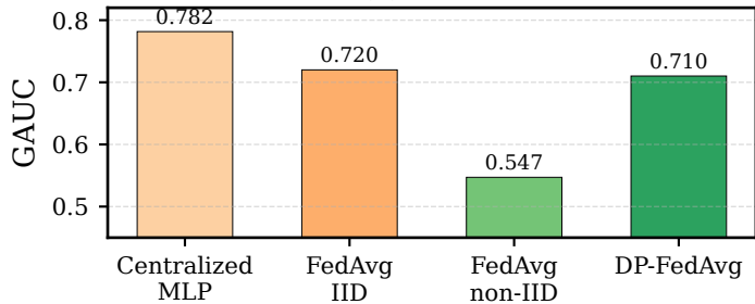
(a) GAUC
