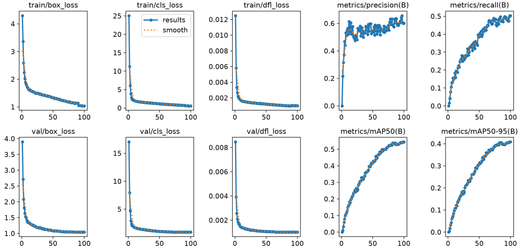
图 3: Stage 1 (YOLO26s 基线) 训练曲线: box_loss、cls_loss 与 mAP@0.5 / mAP@0.5:0.95、Precision / Recall 随 epoch 变化
