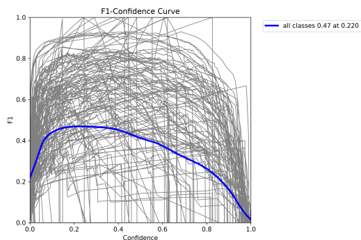
图 6: Stage 1 F1-Confidence 曲线 (各类别 + 全类)
