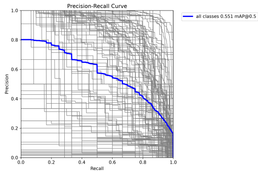
图 11: Stage 2 Precision-Recall 曲线
