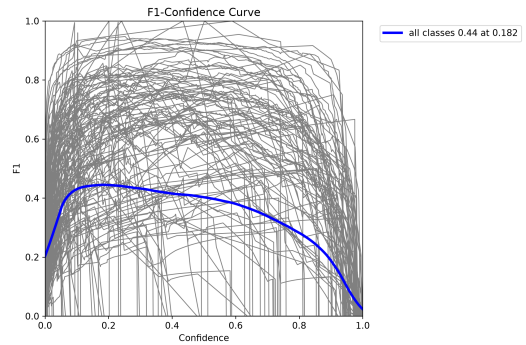
图 12: Stage 2 F1-Confidence 曲线
