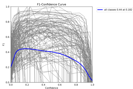
图 12: Stage 2 F1-Confidence 曲线
