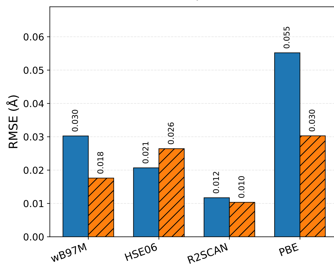
(b) Lattice parameter
