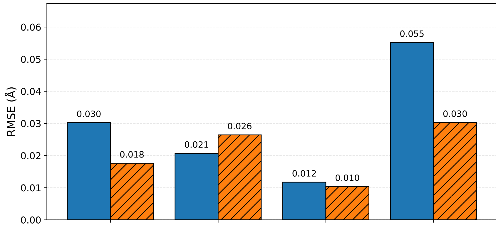
Lattice parameter
