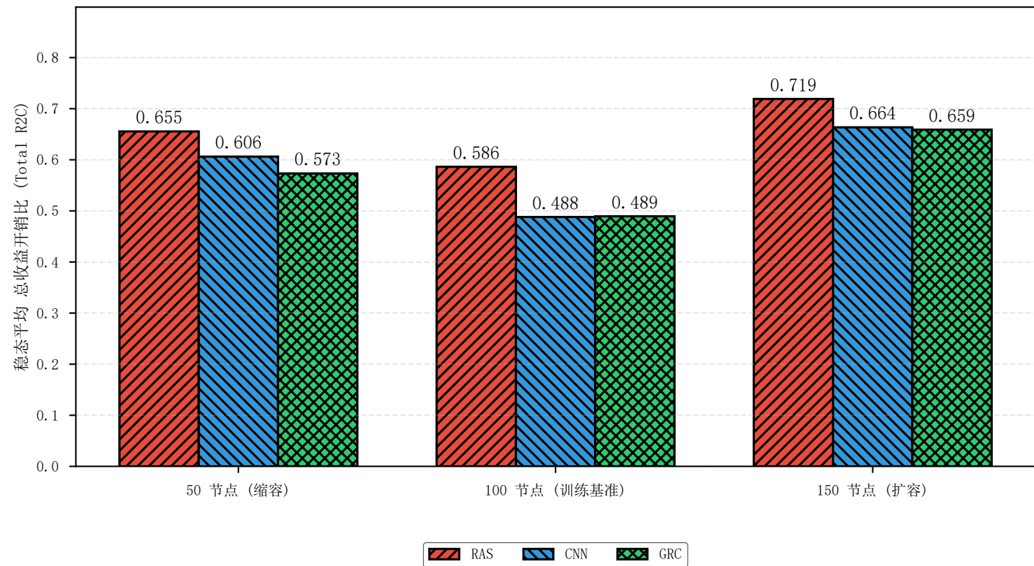
同规模下不同算法的 总收益开销比 (Total R2C) 表现对比
