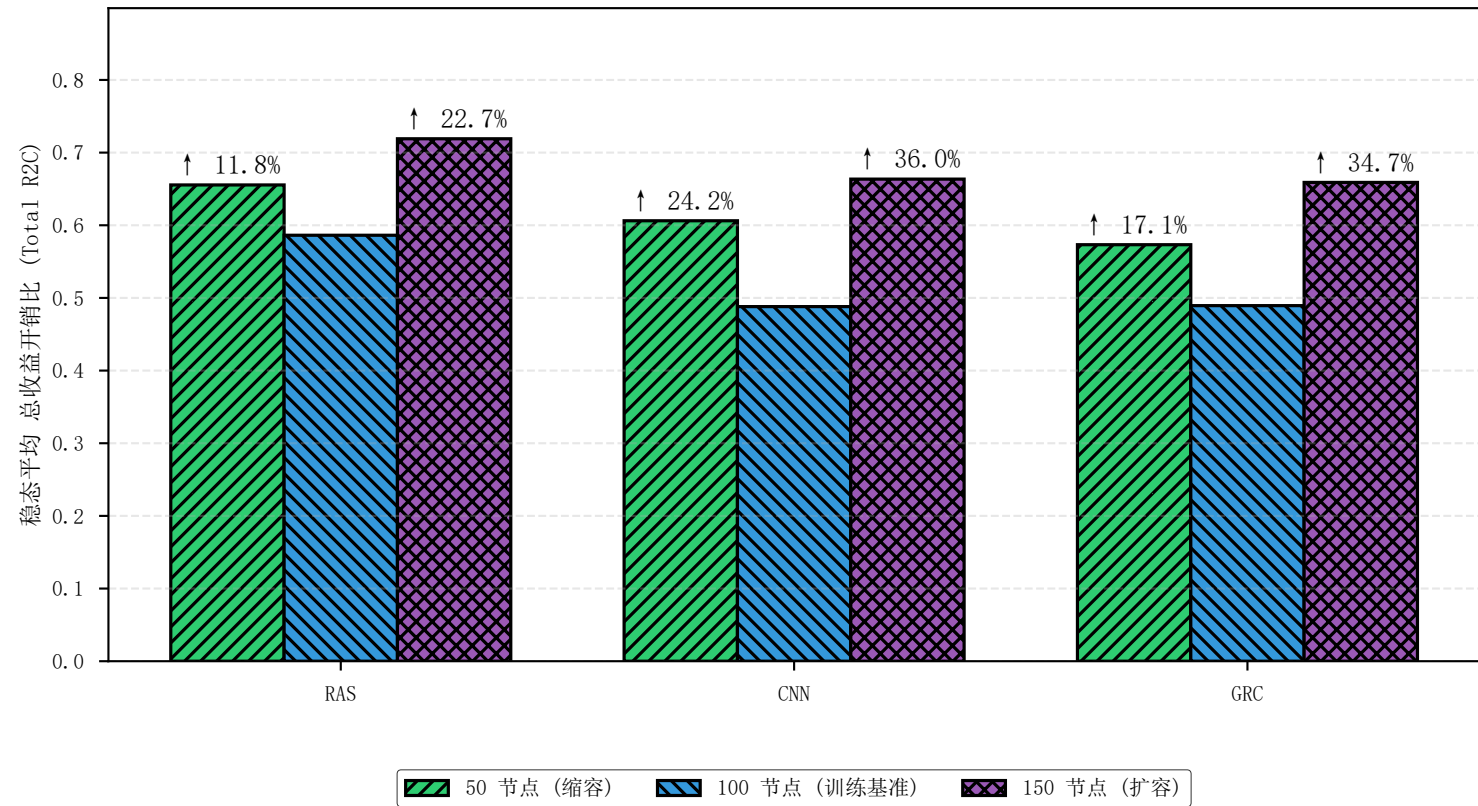
不同网络规模下的 总收益开销比 (Total R2C) 可扩展性分析
