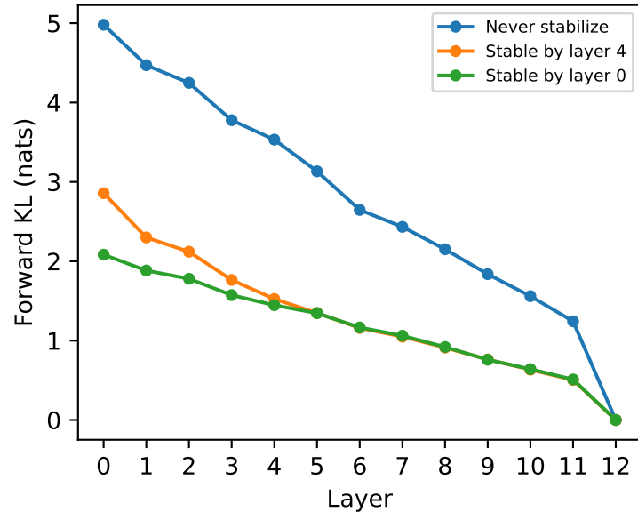
KL divergence to final layer
