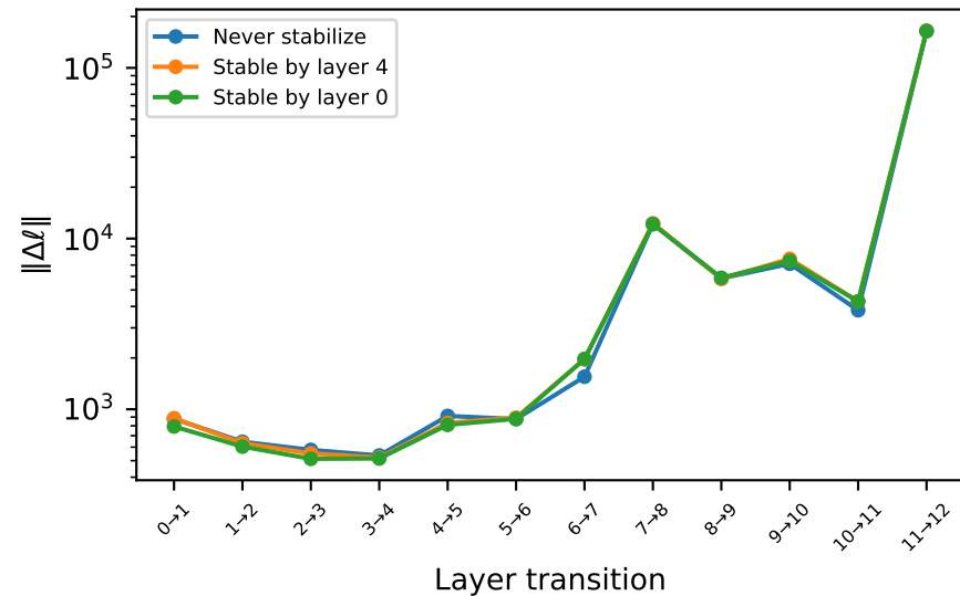
Logit update magnitude
