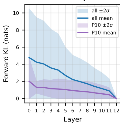
c) Forward KL trajectories
