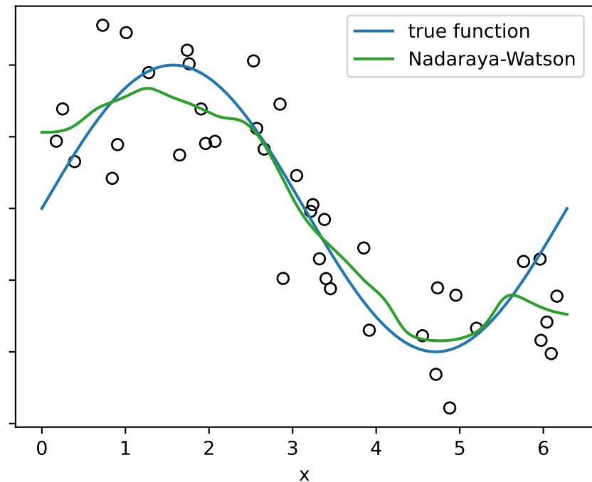
Nadaraya-Watson estimator
