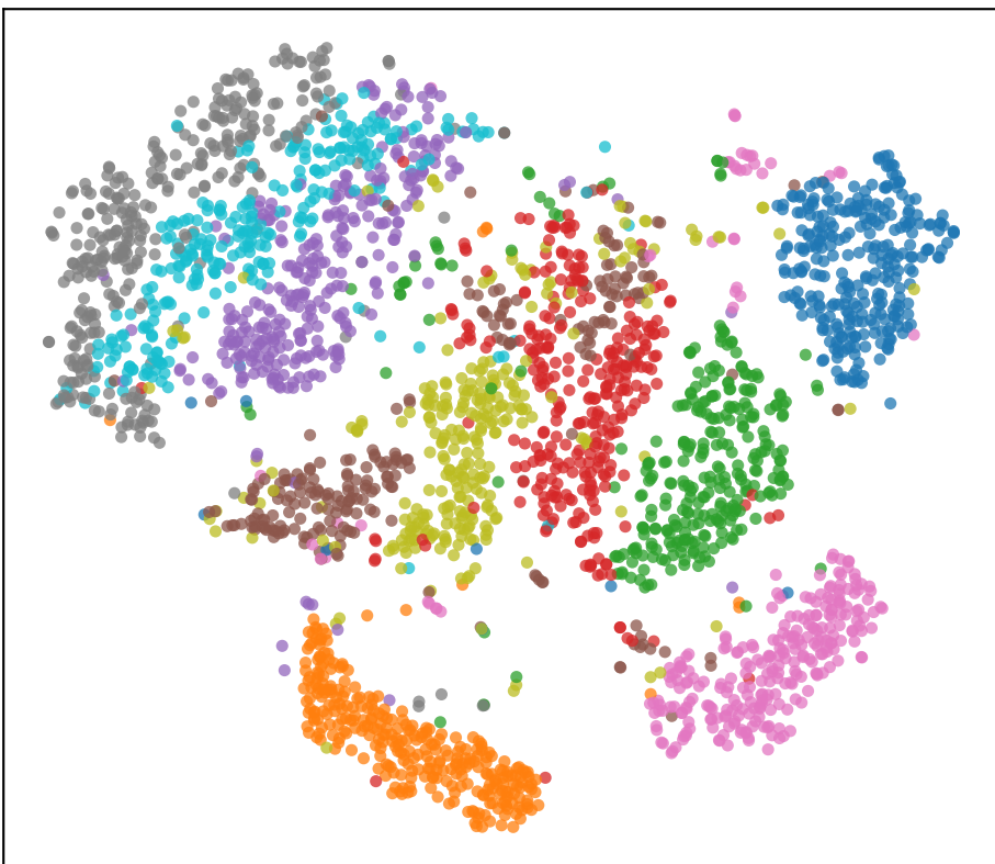
PCA50 + t-SNE
