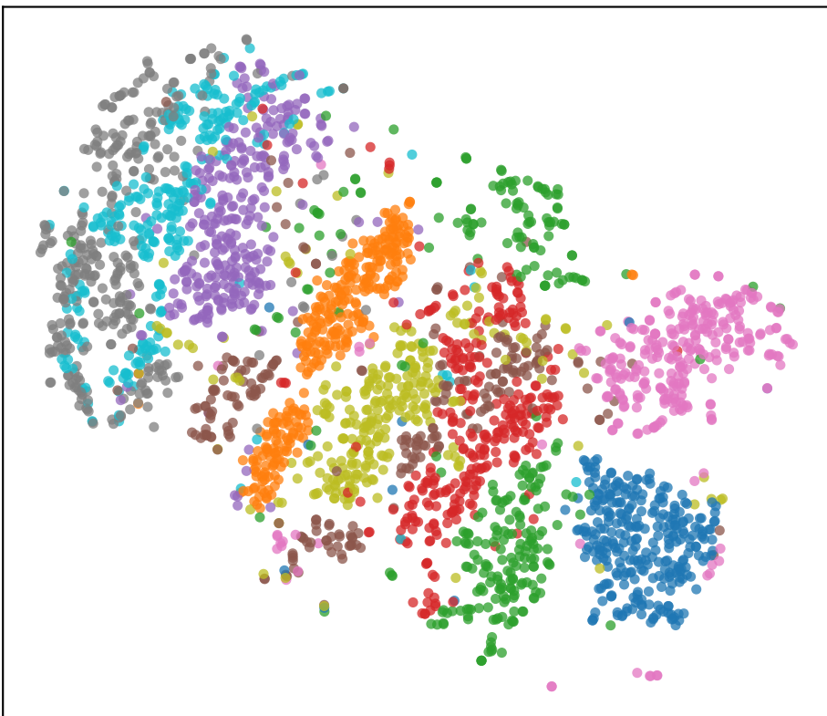
PCA50 + t-SNE
