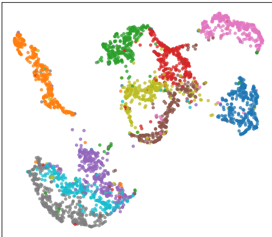
PCA50 + UMAP
