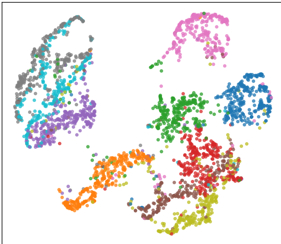
PCA50 + UMAP
