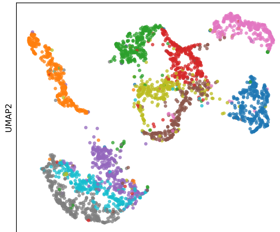
PCA50 + UMAP
