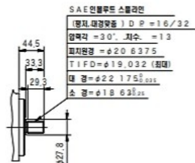
No.11 스프라인 축단형상
