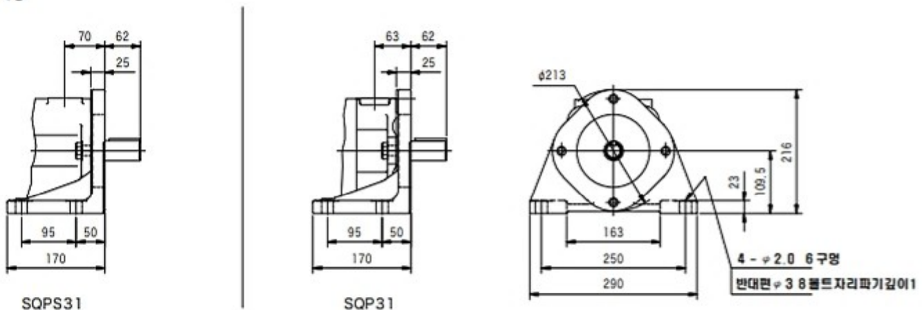
FOOT 접속형
