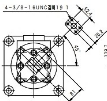
FOOT 접속형
