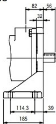
SQPS42
