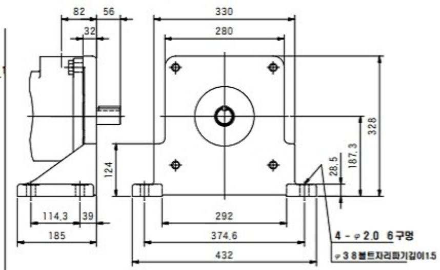
(FOOT 취부)
