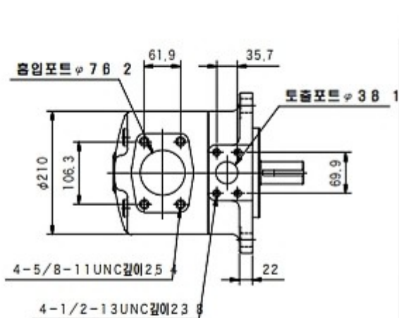
SQP4 (플랜지 취부)
