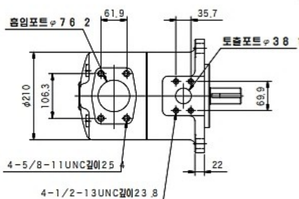
SQPS4 (플랜지 취부)
