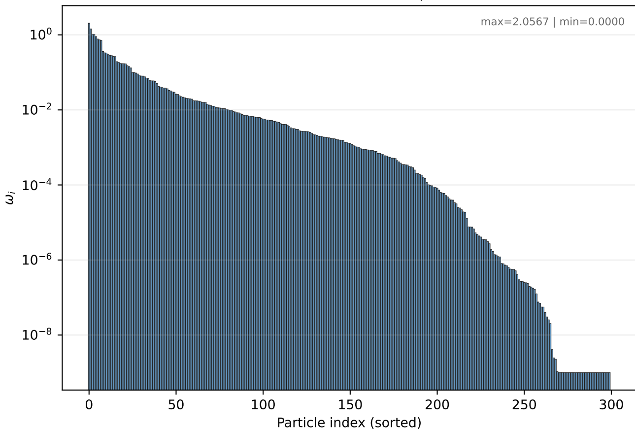
Stochastic CPGD (no BD) (p=300)
