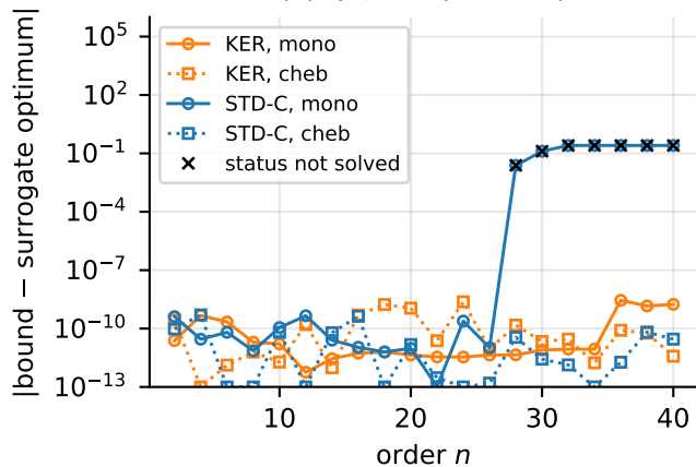
(b) Q1, SCS ( \varepsilon = 10^{-9} )
