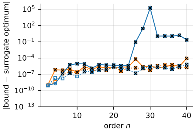
(c) Q1, Clarabel (default)
