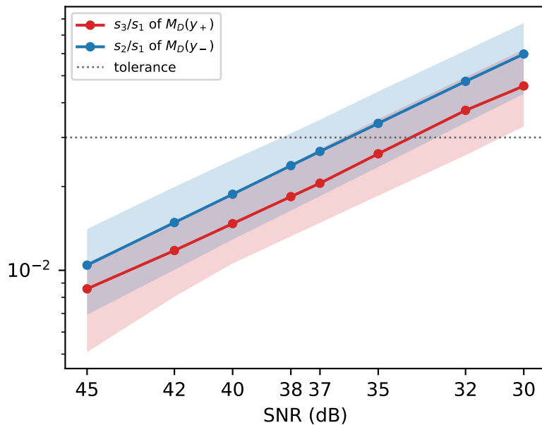
(b) critical singular values
