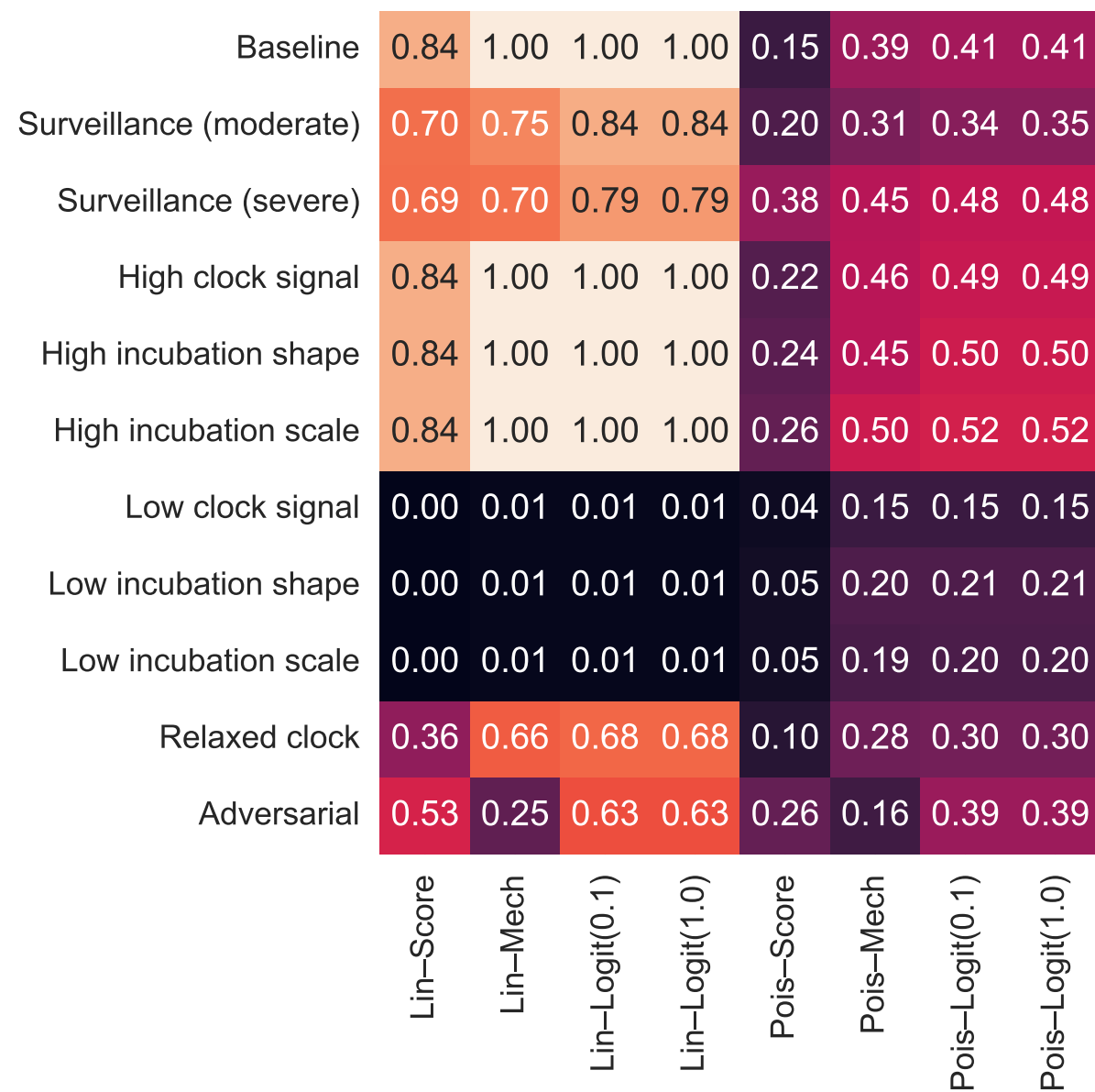
(a) Edge discrimination
