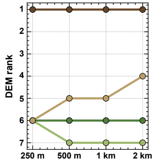
(a) DEM (topographic)
