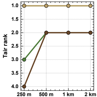
(d) Tair (climate)
