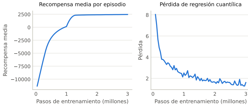
Figura 6.1: Curvas de entrenamiento de la ejecución MAIN. Fuente: elaboración propia a partir de plots/tensorboard_scalars/ de MAIN.
