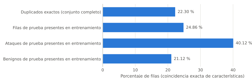
Figura 6.5: Duplicados exactos y fuga entre entrenamiento y prueba en la partición aleatoria fija. Fuente: elaboración propia a partir de runs/validation/duplicate_analysis_seed42.json .
