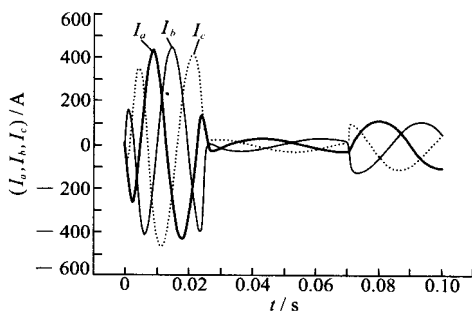
图 5 仿真的三相定子电流波形
