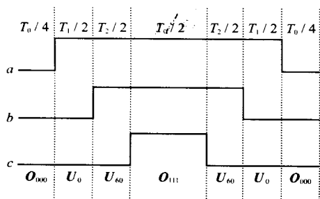
图 3 软开关方案 U_{out} 在 0 \sim 60 内的开关顺序
