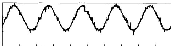
图 7 稳态时的电流实验实测波形
