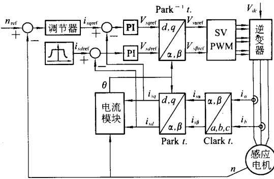
图 2 SVPWM 控制方法框图
