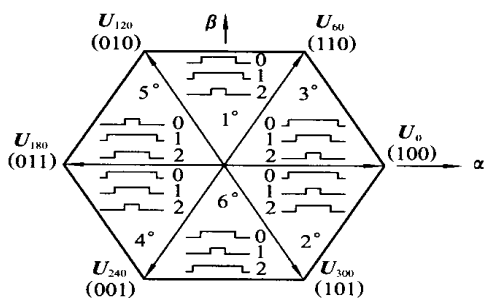
图 4 各区域的 PWM 波形
