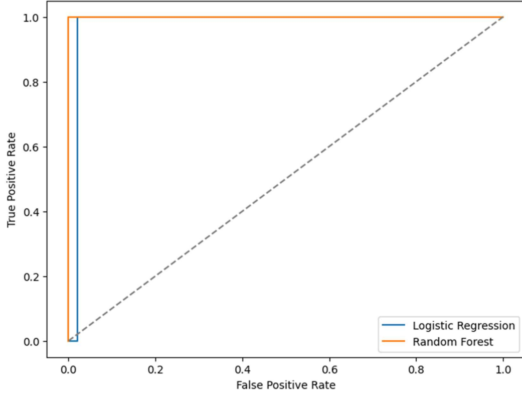
ROC Curve Karşılaştırması
