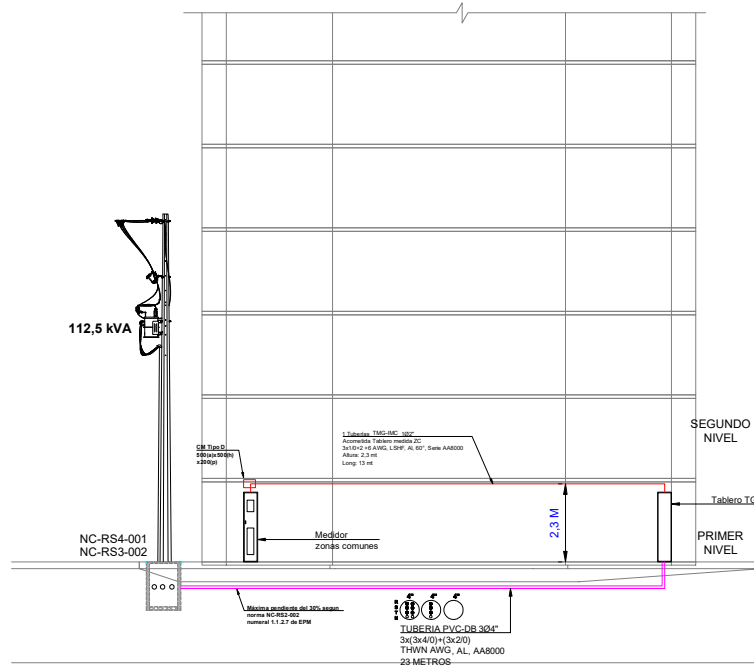
DISTANCIA DE SEGURIDAD (VISTA FRONTAL) ESCALA 1:125
