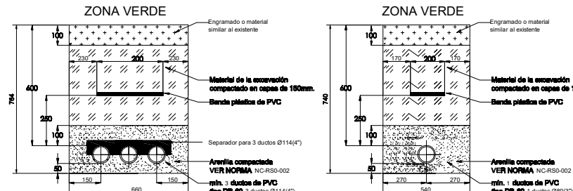
CANALIZACIONES SUBTERRANEAS VER NORMAS RS0-002, RS1-003, RS1-004
