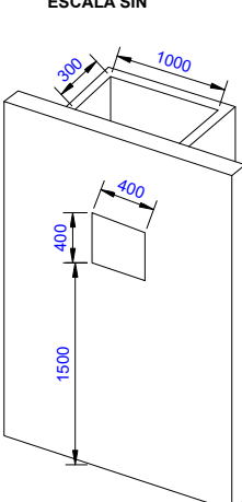
VENTANA DE INSPECCION ESCALA SIN
