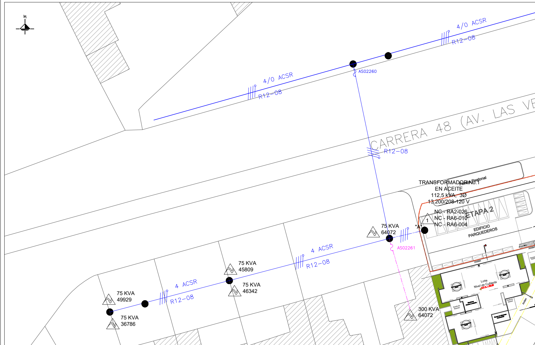
LOCALIZACIÓN Y REDES EN MEDIA TENSION ESCALA 1:300
