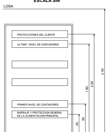
VISTA FRONTAL DE GABINETES DE MEDIDORES PISOS 3, 8, 13, 18, 23 ESCALA SIN
