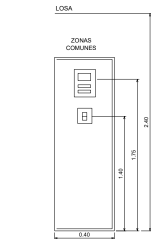
VISTA FRONTAL DE GABINETES DE MEDIDOR DE ZONAS COMUNES ESCALA SIN
