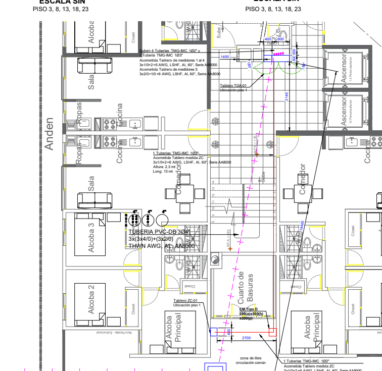
REDES EN BAJA TENSION ESCALA 1:100
