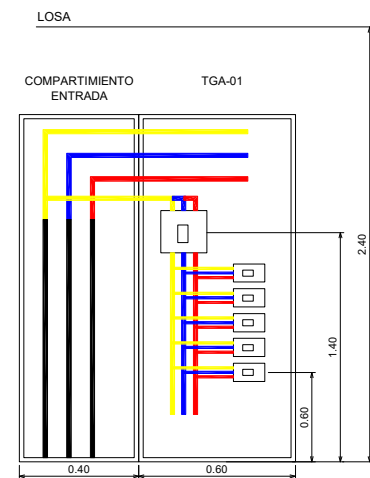
VISTA FRONTAL DE GABINETES ESCALA SIN
