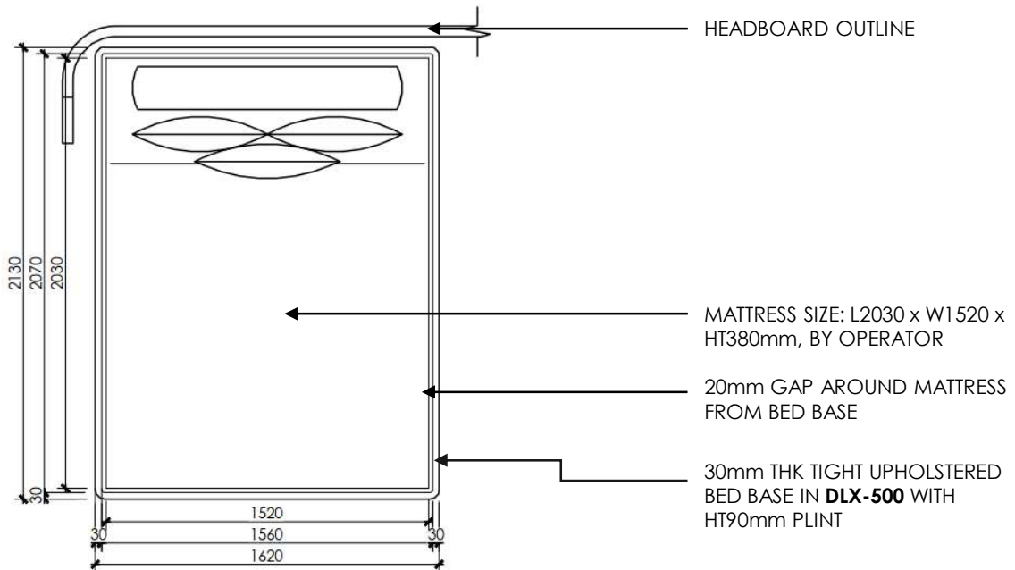
TOP VIEW SCALE: 1:30
