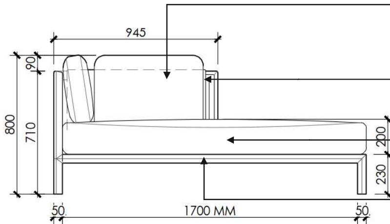
FRONT VIEW SCALE: 1:20
