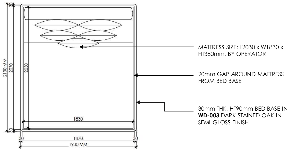
TOP VIEW SCALE: 1:30
