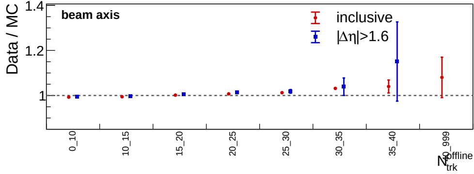
(b) Data/MC ratios
