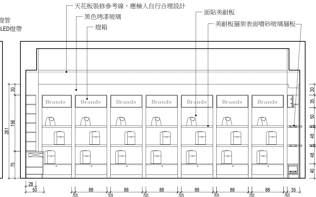
D立面圖
