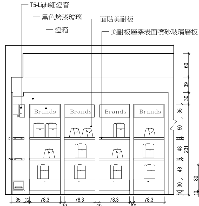
B1立面圖
