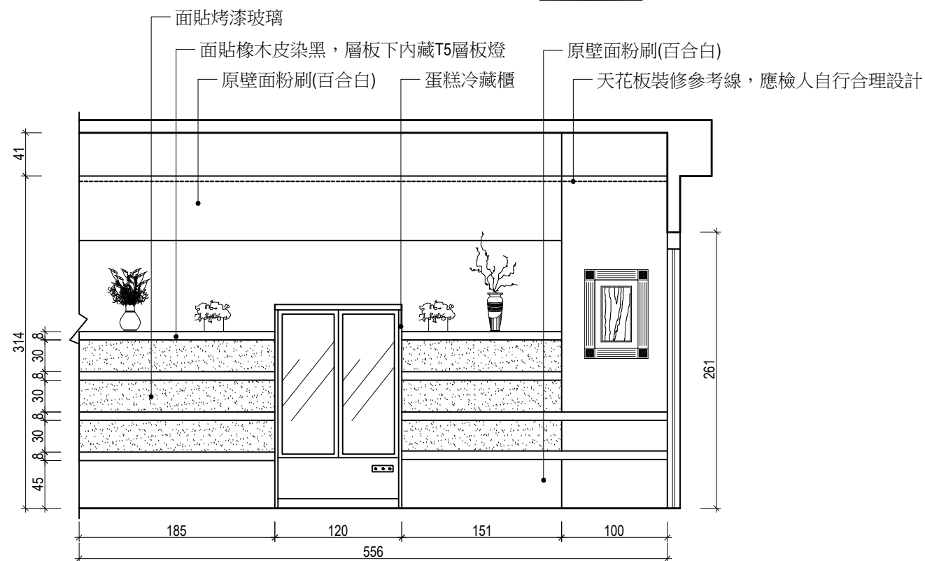
A立面圖
