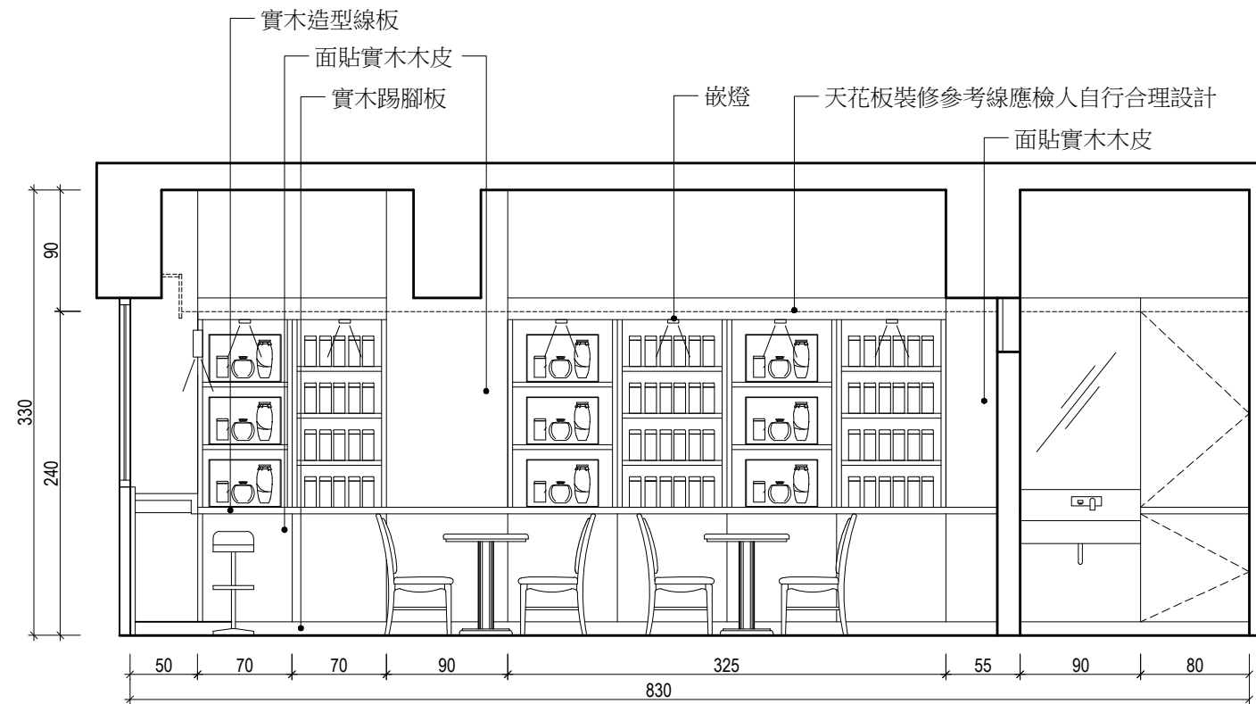
A立面圖
