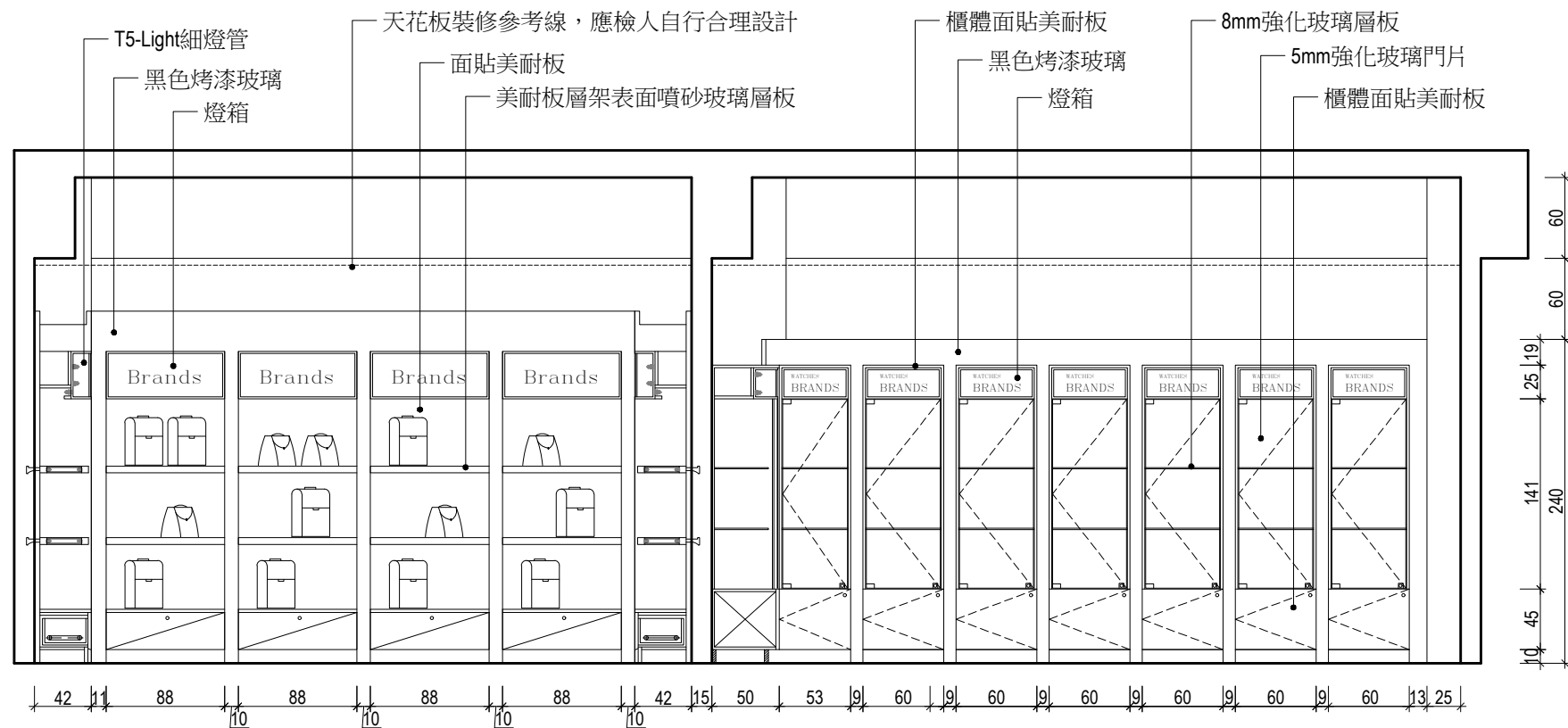
A立面圖
