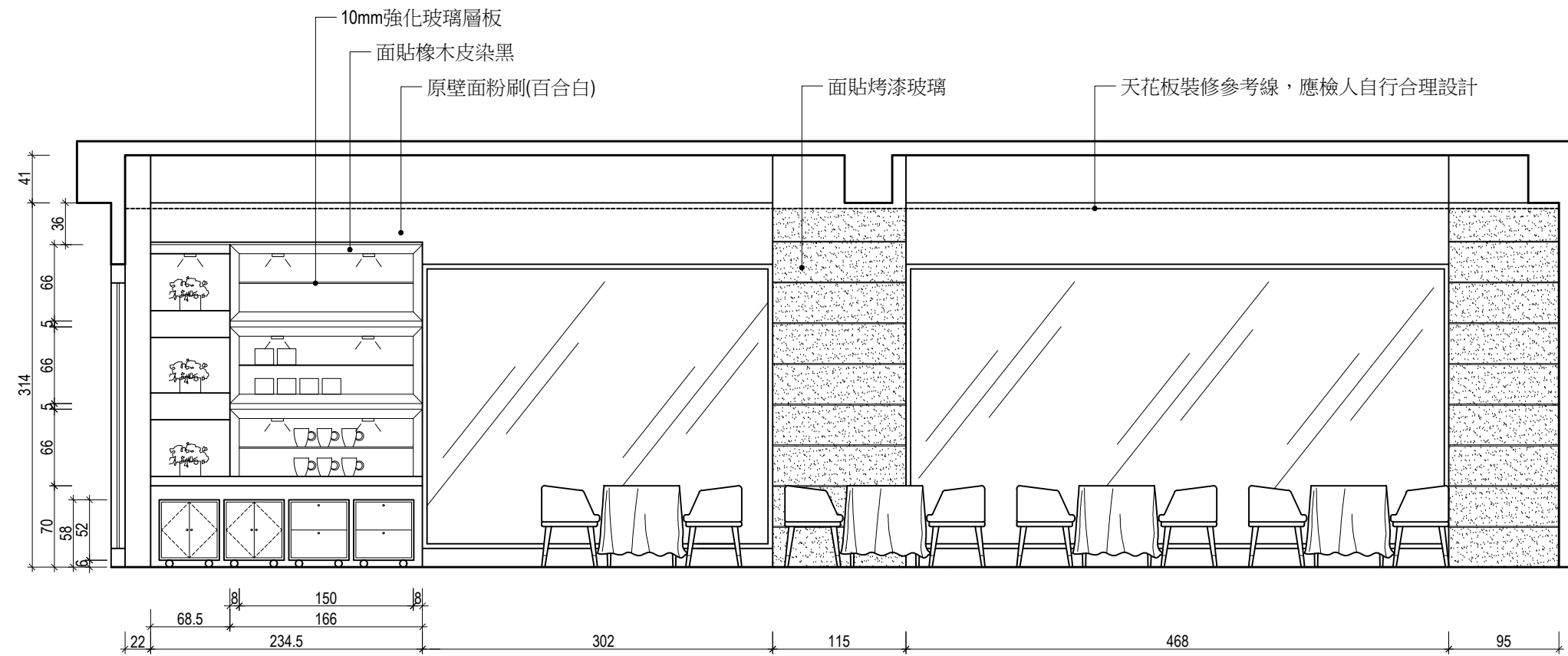
A立面圖
