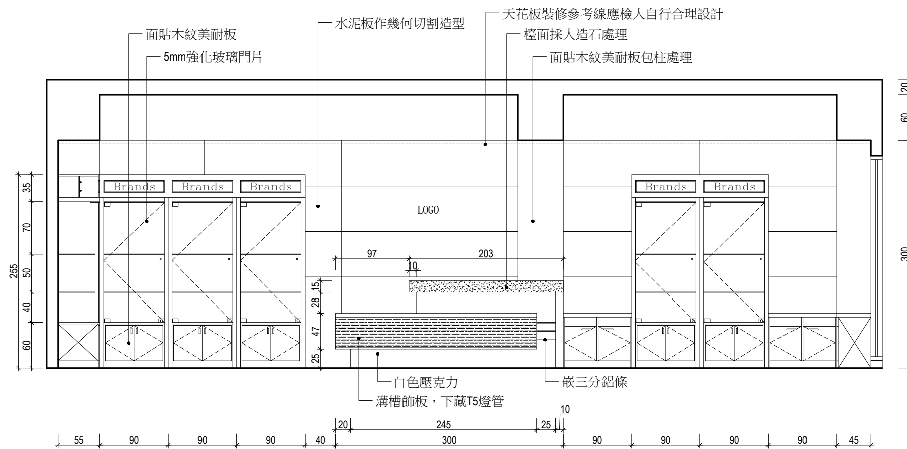
C立面圖
