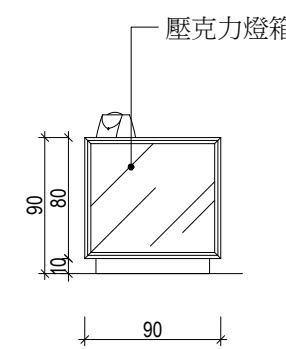
側視圖
