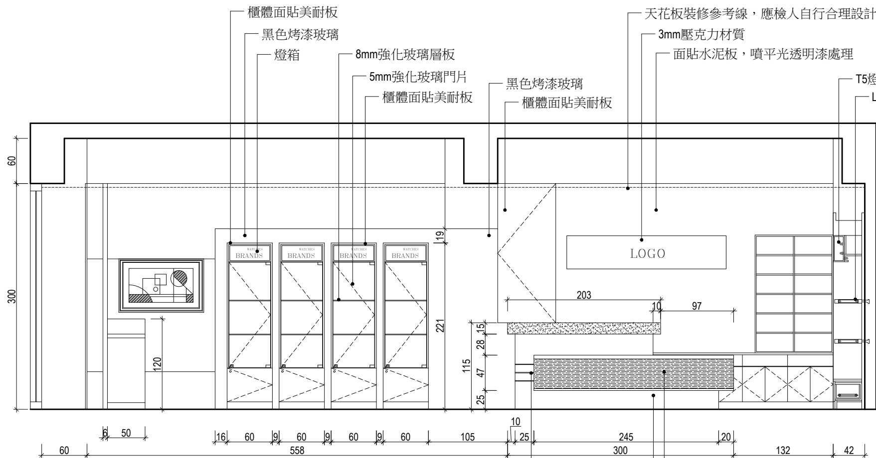
C立面圖
