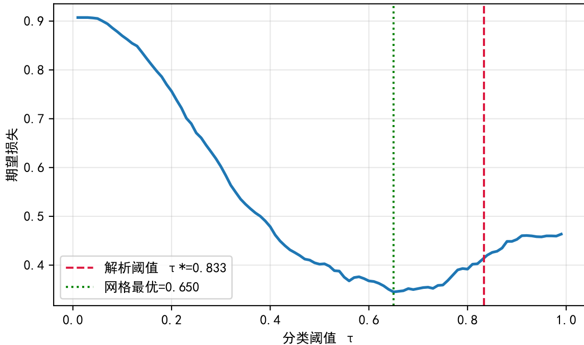
损失矩阵 L_{FN}=5.0 , L_{FP}=1.0
