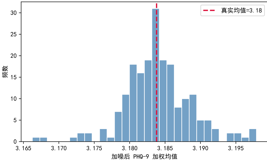
Laplace 机制 ( \epsilon=1.0 )
