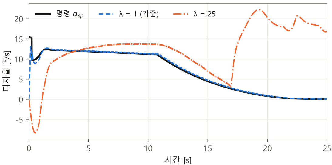
(나) 유도 페루프 — 같은 \lambda 가 명령 추종을 잃고 스스로 당긴다
