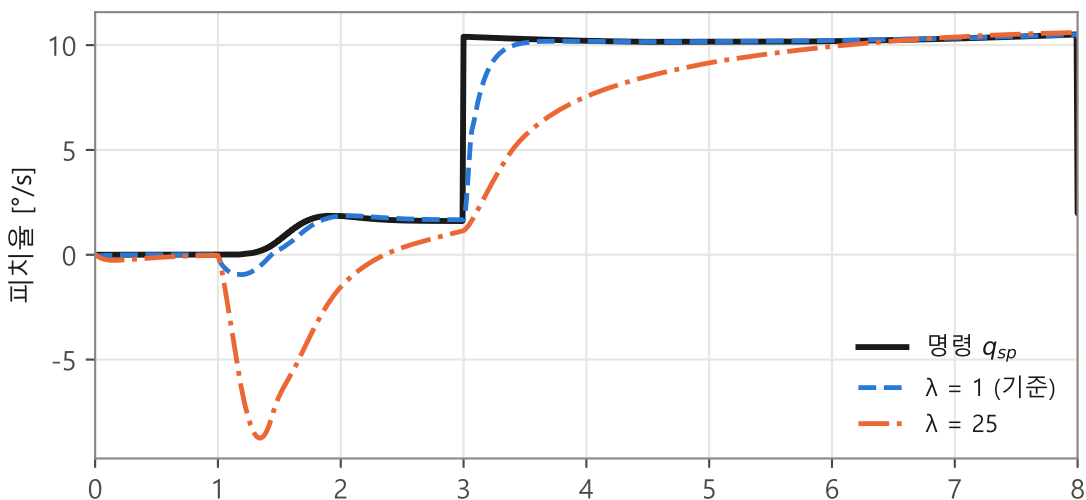
(가) 고정 계단 명령 — \lambda 가 크면 뒤쳐진다
