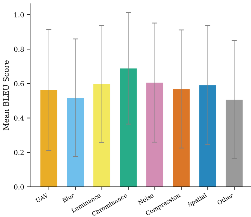
BLEU (Precision)
