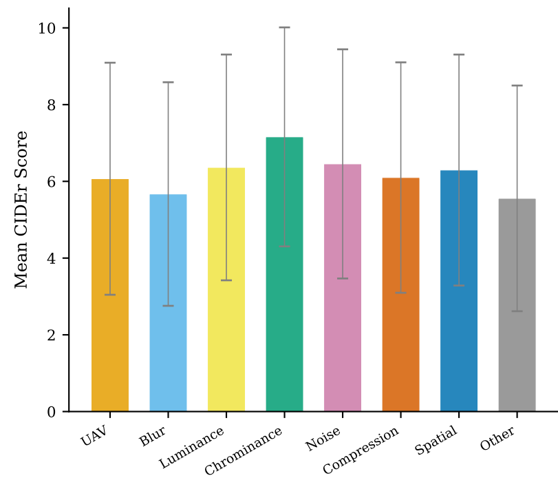
CIDEr (Semantic)
