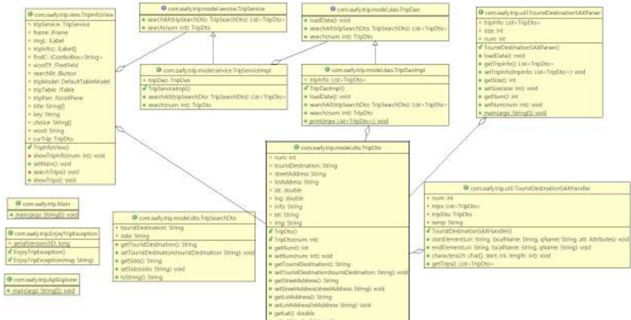
<그림 5> 클래스 다이어그램
