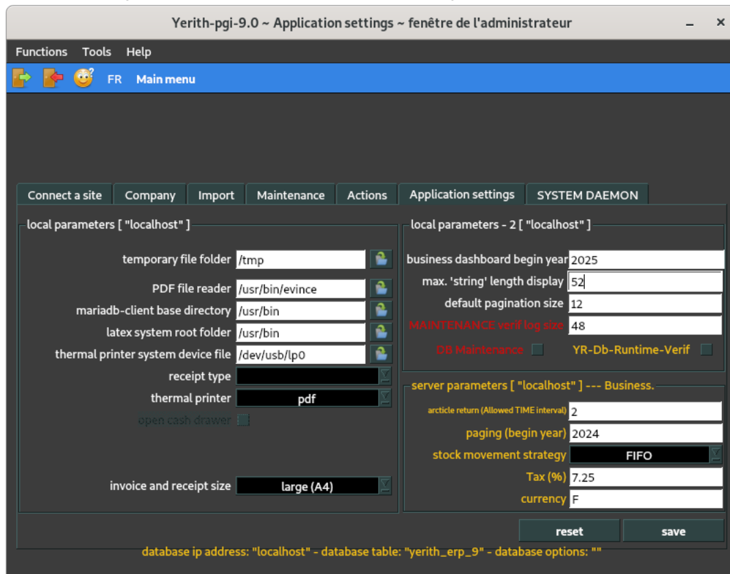
Figure 3.2: La fenêtre de paramétrage du PGI yeritherp.
