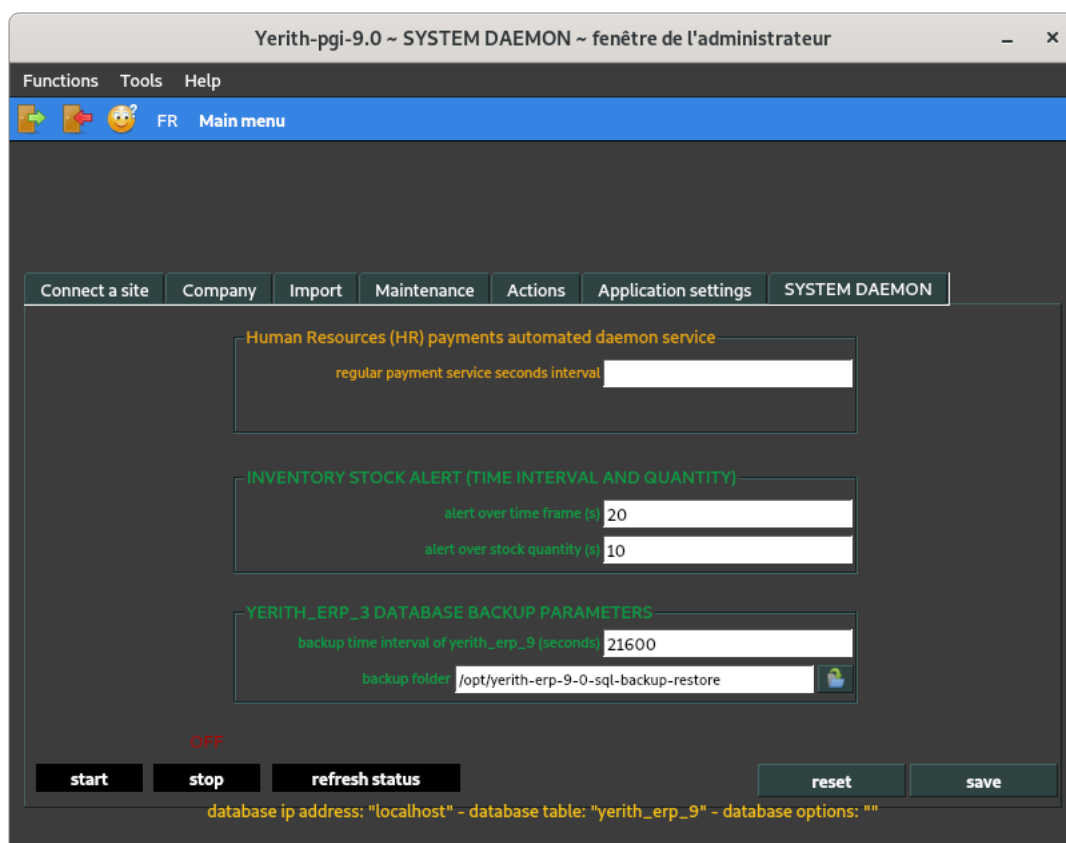
Figure 3.3: La fenêtre de paramétrage du système d'alertes, et du système de sauvegarde automatisée.
