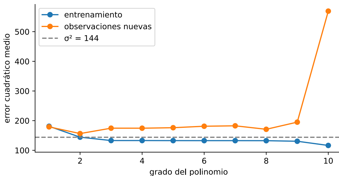
Figura 1: Simulación con mecanismo conocido (demanda curva según precio, \sigma = 12 ). El error en entrenamiento disminuye con el grado; en datos nuevos aparece el compromiso sesgo–varianza. La línea discontinua es \sigma^2 .
