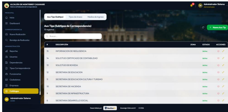
Figura 12. Módulo Catálogos
