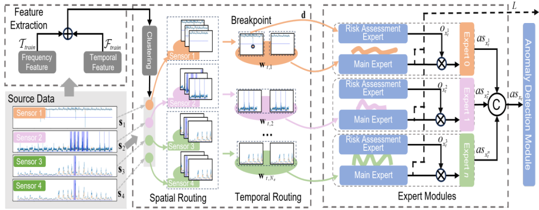
图 19: 混合专家的多传感器时序异常检测框架
