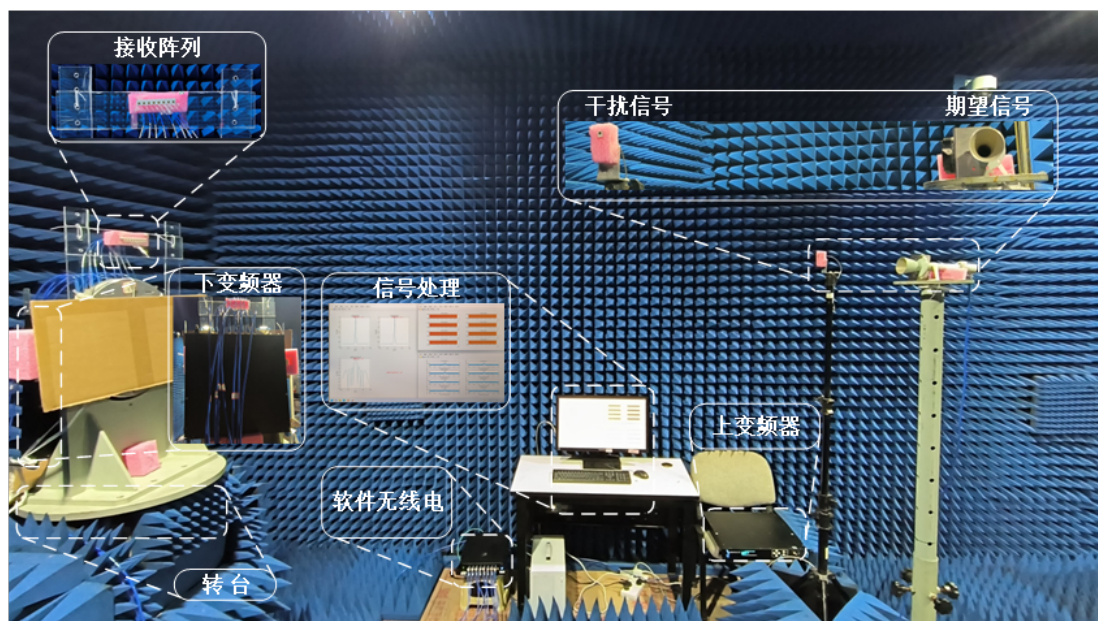
图 24: 无线电测向系统实拍图
