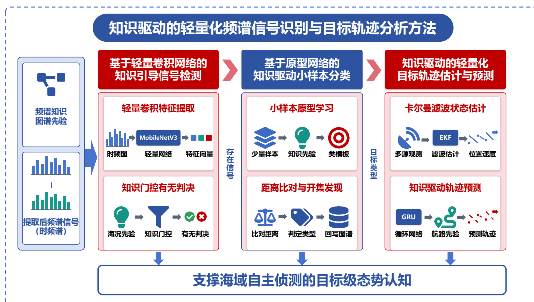
图 14: 知识驱动的轻量化频谱信号识别与目标轨迹分析方法
