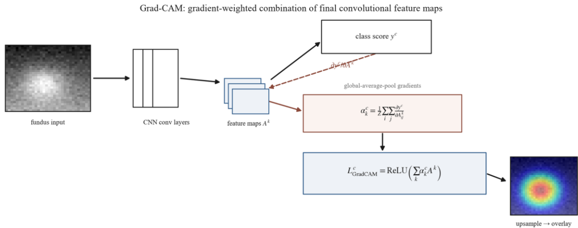
Сурет 2.7 – Соңғы қабаттың белгі карталарын градиентпен салмақтап біріктіру
