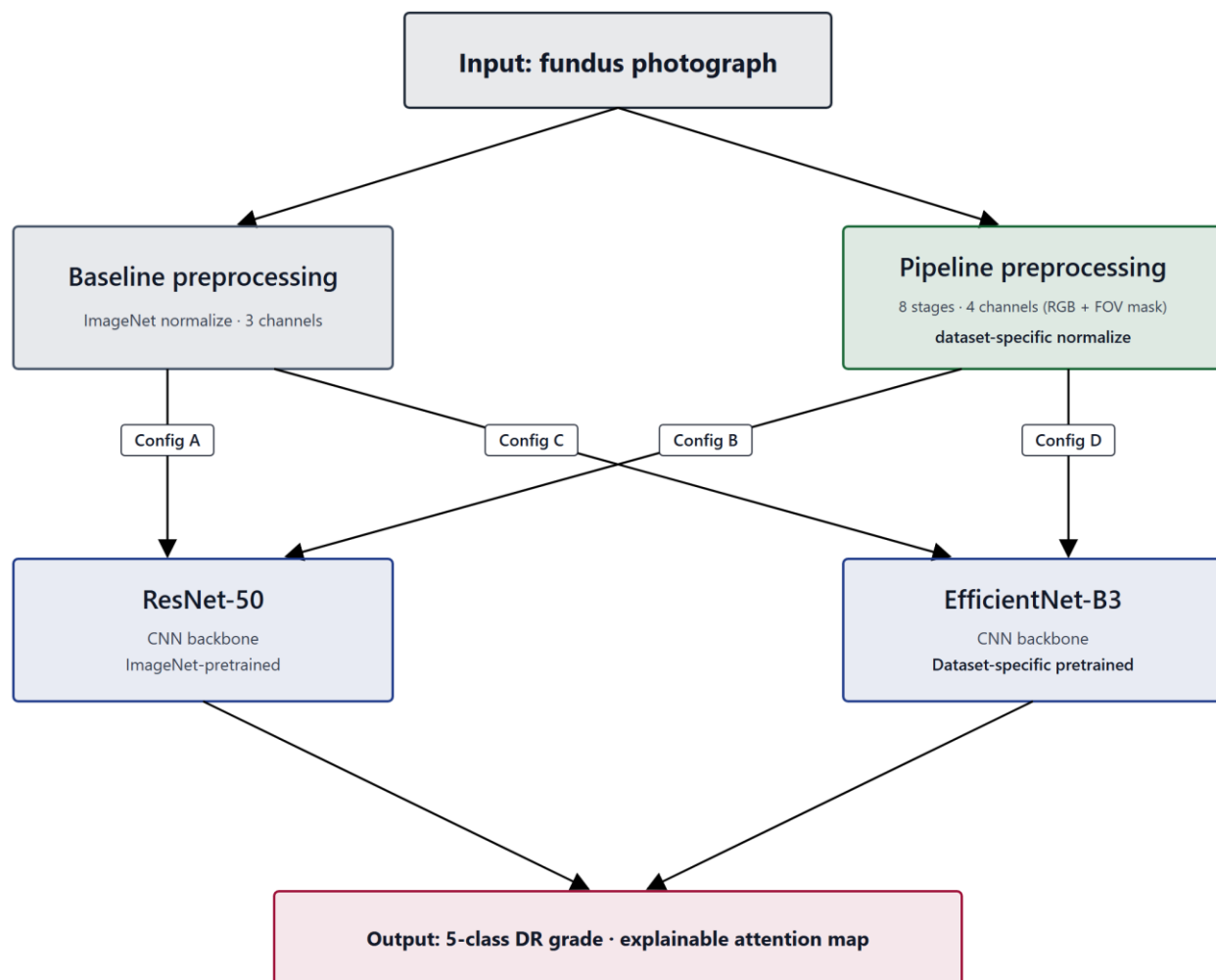
Сурет 3.12 – ResNet-50 / EfficientNet-B3 backbone архитектурасы
