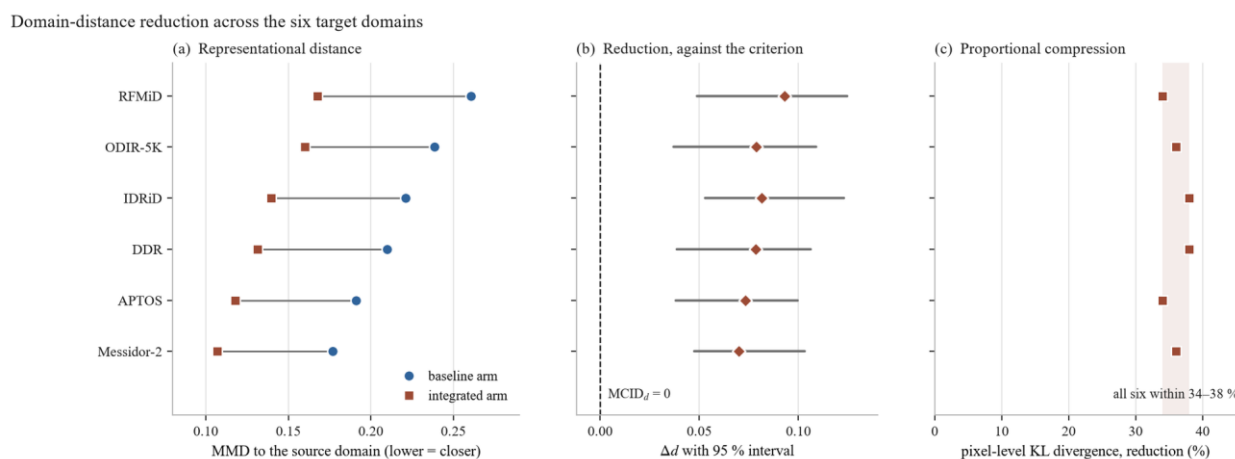
Сурет 4.4 – Алты нысаналы домен бойынша домен қашықтығының азаюы, екі өлшем бойынша. (a) әр арнадағы репрезентациялық қашықтық, бастапқы алыстығы бойынша реттелген; (b) азаю өзінің 95 % интервалымен MCID d = 0-ге қарсы – вердиктті алып жүретін панель; (c) пиксел деңгейіндегі азаю пайызбен, өзі түсетін жолаққа қарсы. (a) панелі әр арнаның өз белгілер кеңістігінде өлшенген, сондықтан екі баған бір ортақ кеңістіктегі қашықтықтар емес, әр модельдегі салыстырмалы алыстық; (c) панелі – қосалқы, ақпараттық өлшем әрі вердикттің бөлігі емес. Сурет тек бағыт пен дәйектілікті көрсетеді – ешбір панель қашықтық азаюын тасымалдау өсімімен жұптастырмайды, әрі ешқайсысы азаю шамасы өсім шамасын болжайды деген тұжырымды қолдауға арналмаған
