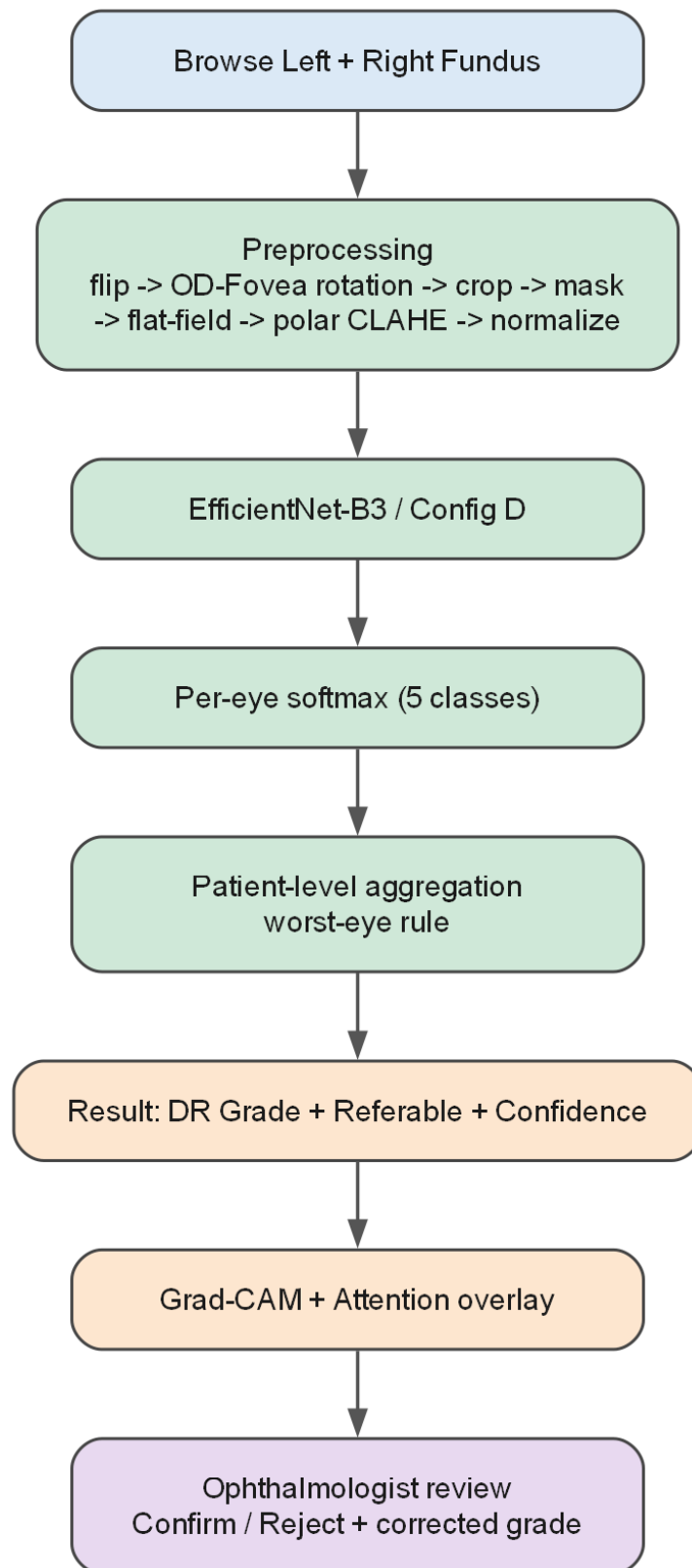
Сурет 3.2 – End-to-end модель блок-схемасы, model = preprocessing + CNN
