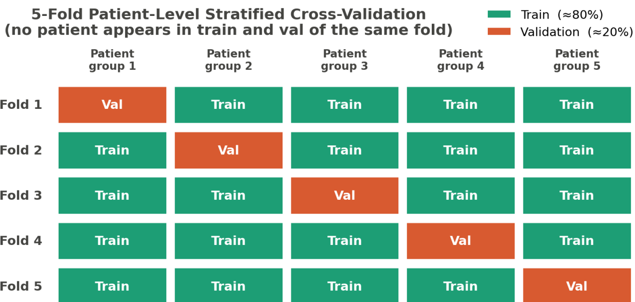
Сурет 3.14 – 5-fold пациент-деңгейлі cross-validation бөлуі
