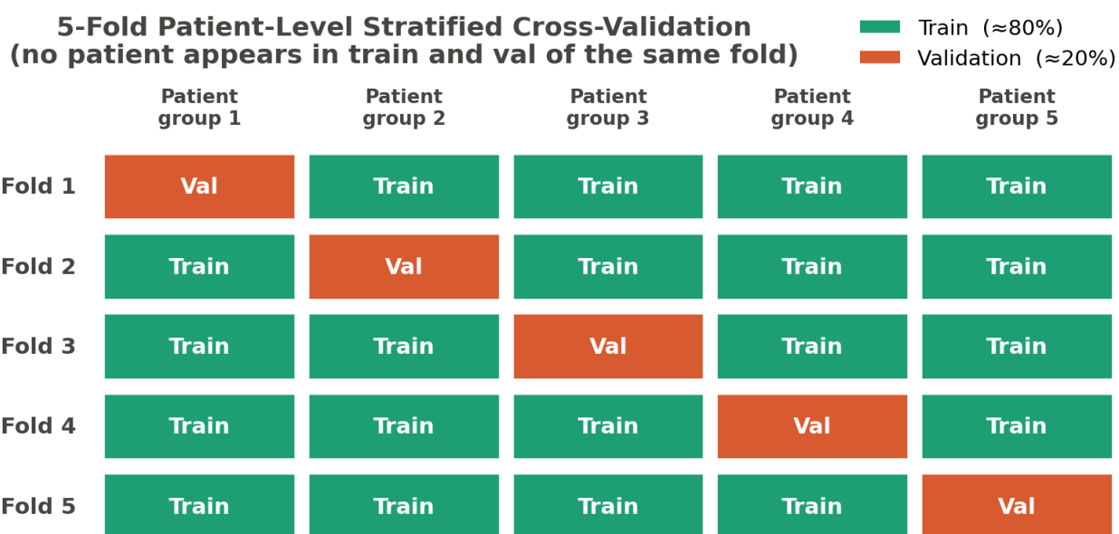
Сурет 3.13 – 5-fold пациент-деңгейлі cross-validation бөлуі
